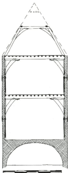
Dwarsdoorsnede van Langebrug 55. Reconstructie door Edwin Orsel, naar opmeting door Marlies van der Meijden.
