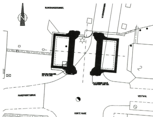
Situatietekening van de funderingen van de Marepoort, ingemeten in april 2002.
