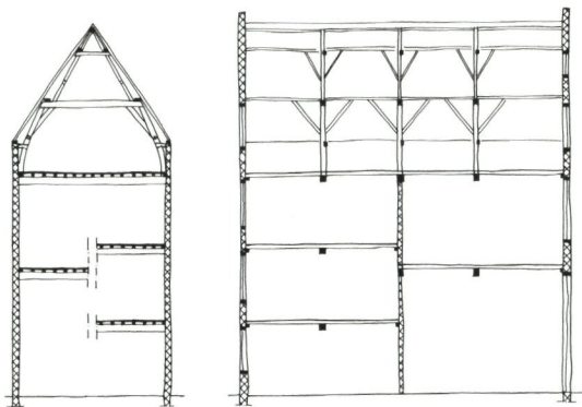
Doorsneden van Donkersteeg 5. Reconstructie door Edwin Orsel.
