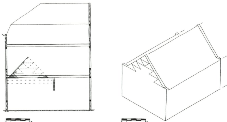
Zuidsingel 34: documentatie van de linkerzijgevel en axonometrie. Tekeningen door Edwin Orsel.
