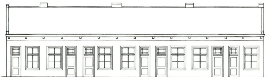
De voorgevels van de kamerwoningen. Reconstructie door Edwin Orsel.
