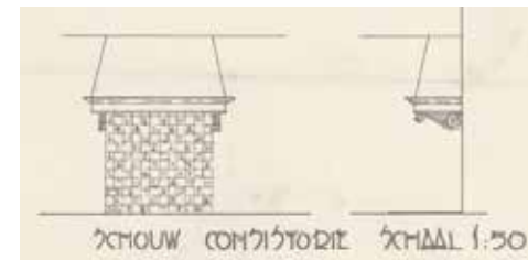
Ontwerptekening consistorie door W. Fontein, 1928 (detail). Erfgoed Leiden en Omstreken.
