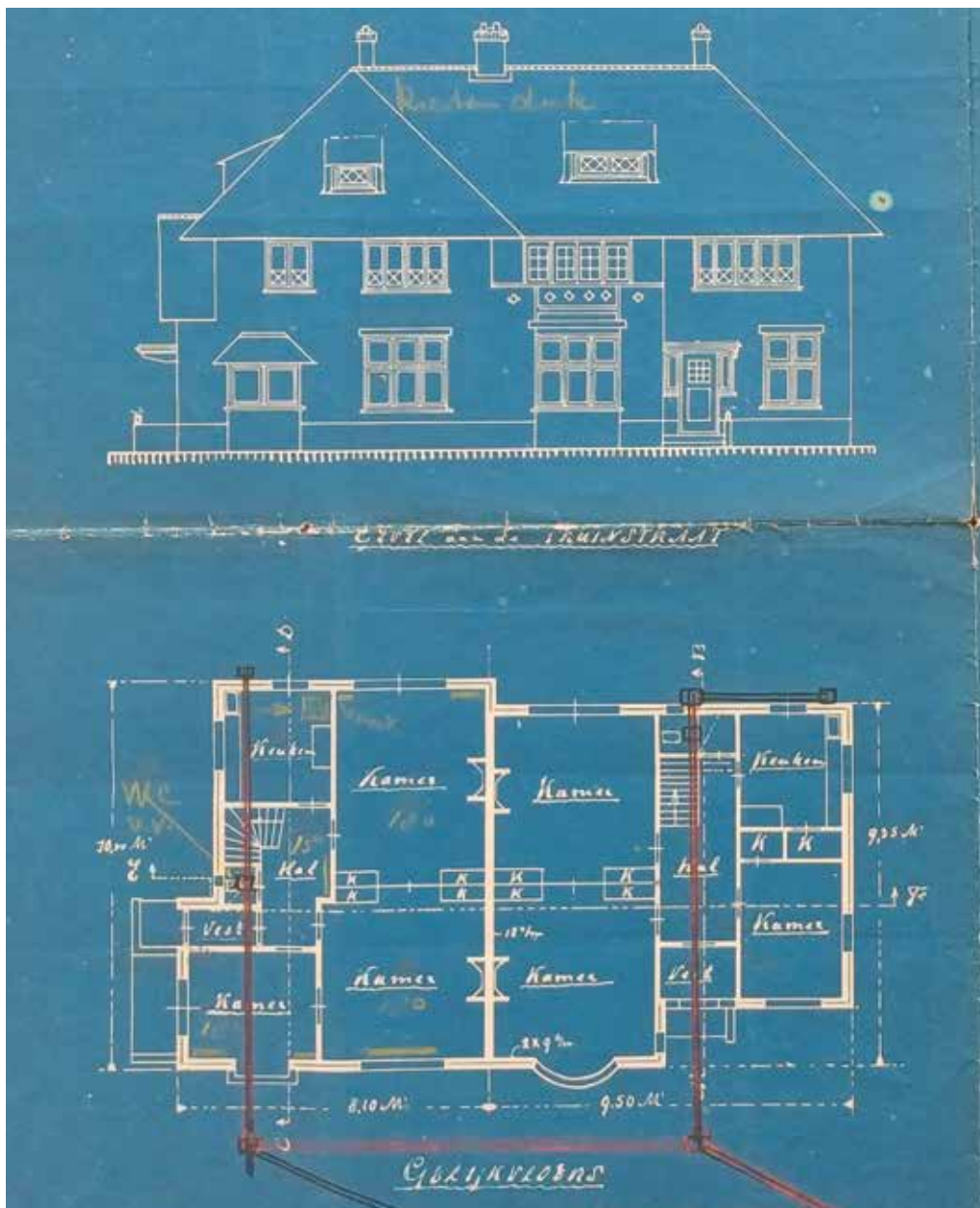
Tekening van het dubbele woonhuis Fruinlaan 5/Cobetstraat 43 in Leiden (detail). ELO, toegang 2033, Archief Reyneveld, inv.nr. 17.
