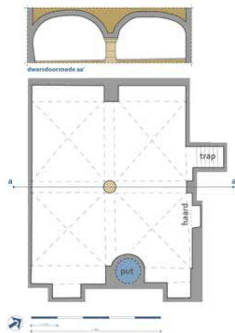
Reconstructie van dwarsdoorsnede (boven) en plattegrond (onder) van het badhuis in de kelder van Diefsteeg 1 / Breestraat 77. Tekening: Erfgoed Leiden en Omstreken.
