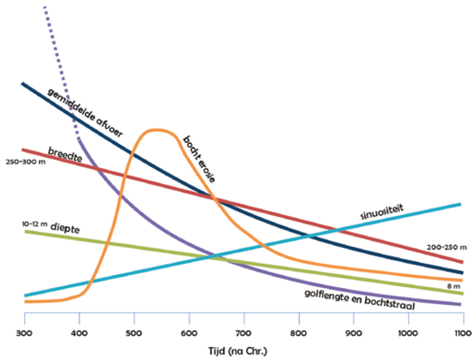
Afbeelding 3. De veranderingen van de dimensies, de afvoer en mate van meanderen tussen de Romeinse tijd en het inactief worden van de Oude Rijn in 1163 na Christus. Grafiek: Antoine Wilbers.
