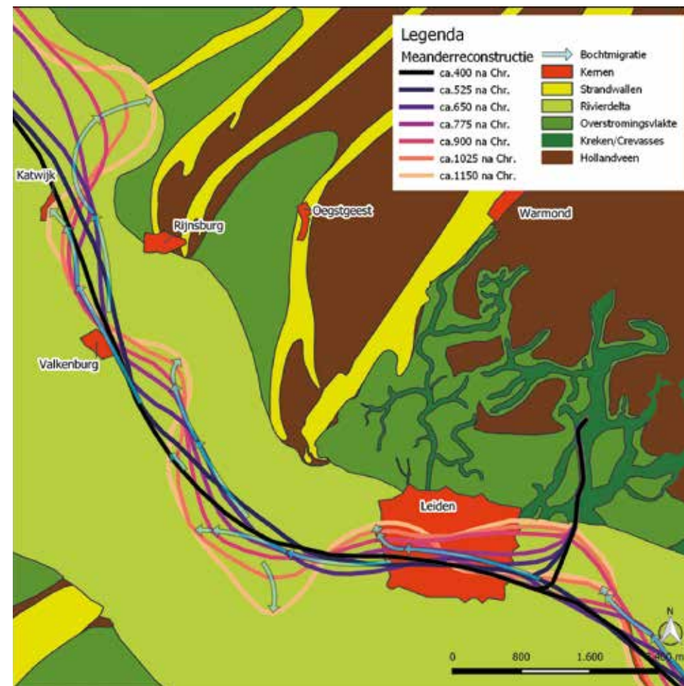
Afbeelding 4. Reconstructie van de meanderbochten uitgaande van de huidige loop van de Oude Rijn. De dateringen zijn geschat, evenals de ligging van de verschillende rivierlopen. Meanderreconstructie: Antoine Wilbers. Kaart: Peter Vos, Michiel van der Meulen, Henk Weerts & Jos Bazelmans, Atlas van Nederland in het Holoceen. Landschap en bewoning vanaf de laatste ijstijd tot nu (Amsterdam, 2018)
