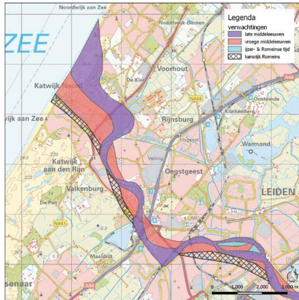
Afbeelding 7. Zones met archeologische verwachtingen als gevolg van het meanderen van de Oude Rijn gedurende de vroege middeleeuwen. Aanduiding zones: Antoine Wilbers.
