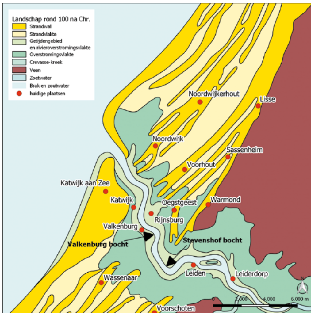
Afbeelding 1. Kaart met paleografische reconstructie van Nederland in de Romeinse tijd rond 100 na Christus, detail met de Valkenburgbocht en de Stevenshofbocht. Gebaseerd op Peter Vos, Michiel van der Meulen, Henk Weerts & Jos Bazelmans, Atlas van Nederland in het Holoceen. Landschap en bewoning vanaf de laatste ijstijd tot nu (Amsterdam, 2018).
