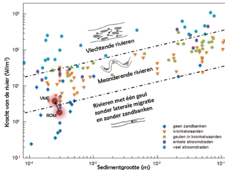
Afbeelding 2. Diagram van rivierpatronen onderscheiden op basis van de kracht van de rivier en het sediment dat vervoerd wordt. Uit het diagram blijkt dat de afname van de afvoer van water door de rivier na de Romeinse tijd een verandering van rivierpatroon veroorzaakt. De verschillende gekleurde punten in het diagram zijn rivieren die over de hele wereld voorkomen. De grote rode stippen geven de Oude Rijn weer. Gebaseerd op Maarten G. Kleinhans & Jan H. van den Berg, 'River channel and bar patterns explained and predicted by an empirical and a physics-based method', Earth Surface Processes and Landforms, 36 (2011) 721-738.
