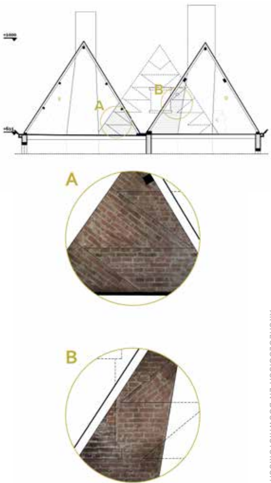
Boven: Doorsnede van het achterhuis van Rapenburg 49 met daarop aangegeven de gevonden bouwsporen. Opmeting met total station in combinatie met fotorectificatie: Pieter-Jan de Vos, Erfgoed Leiden en Omstreken. Sporen A en B: zie afbeelding onder. Onder: Foto's van bouwsporen A en B, aangetroffen in de linker zijgevels ter hoogte van de kapconstructie. Foto: Pieter-Jan de Vos, Erfgoed Leiden en Omstreken.
