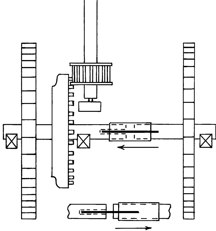
Het inwendige van de molen met twee schepraderen. Horizontaal de uit twee delen bestaande wateras met van links naar rechts: het brede scheprad, waterwiel, ijzeren pen met verschuifbare houten koker en het smalle scheprad. In het midden verticaal naar boven gericht de roterende, door de wieken aangedreven koningsspil met schijffloop. De ontkoppelde situatie is ook afgebeeld. Tekening Wim Zalm, 2020.
