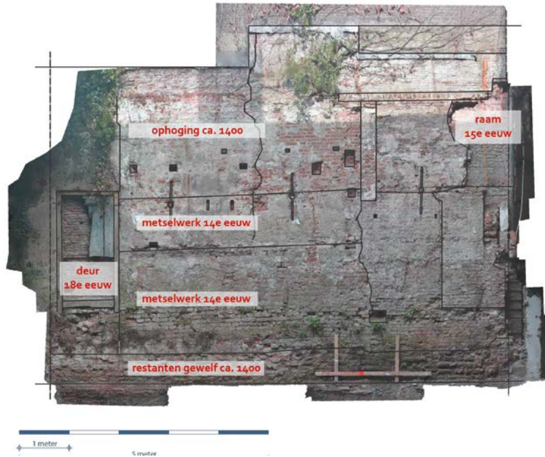
Orthofoto (geometrisch gecorrigeerde foto) van de rechter zijgevel waarop verschillende bouwsporen zijn aangegeven. De muur is deels gesloopt in 2019. Foto: Erfgoed Leiden en Omstreken.
